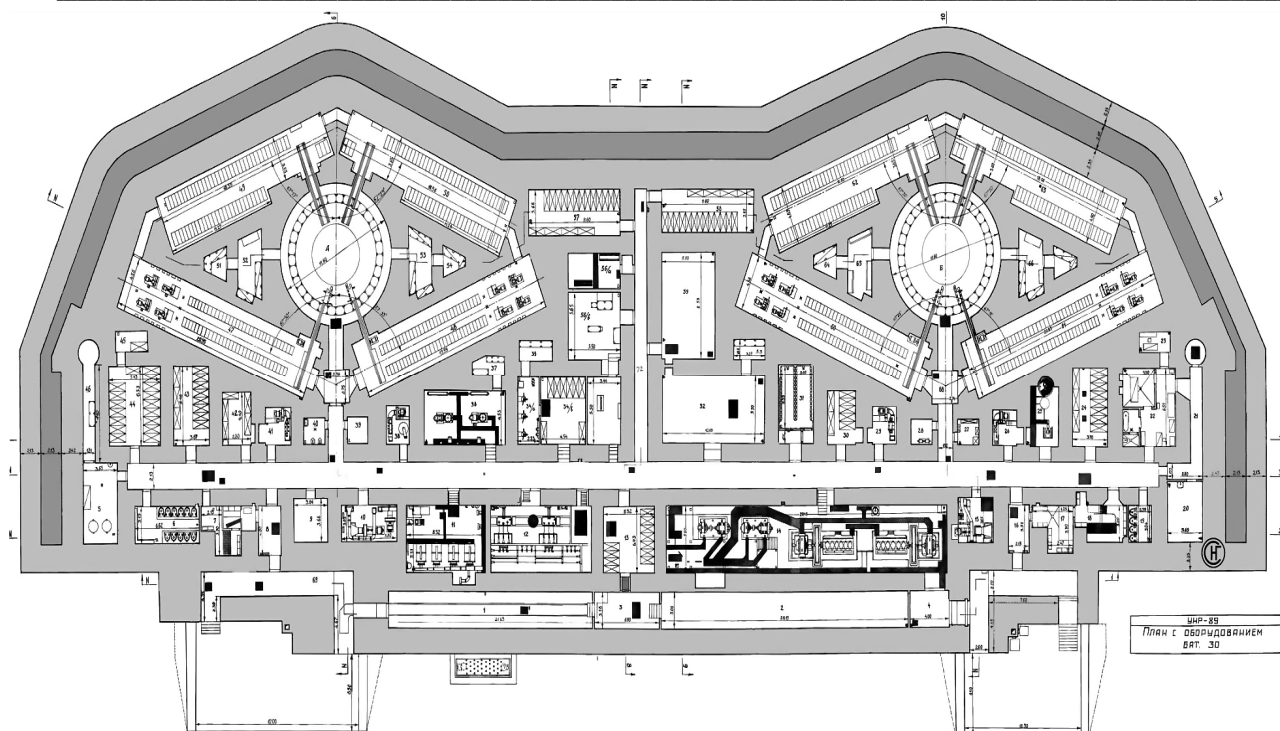
Рис. 1. Экспликация помещений 30-й батареи
