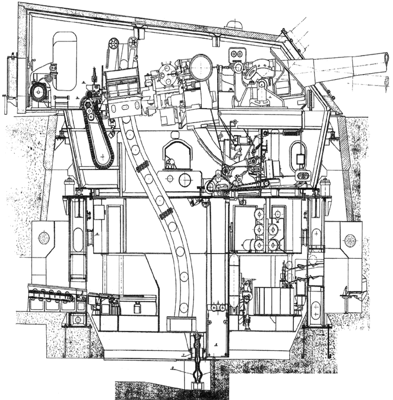
Рис. 2. Схематический разрез башенной установки МБ-2-12ФМ
