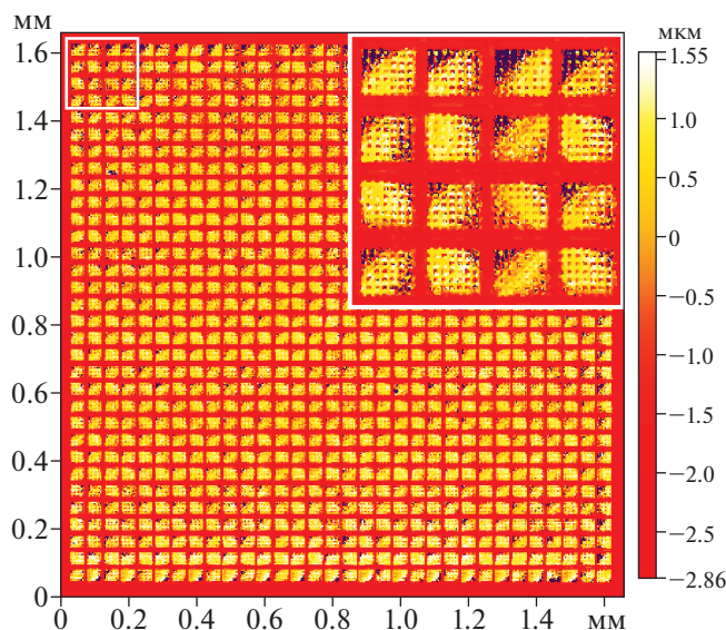
Рис. 2. Оптическое изображение 1738×1717 точек матрицы МЗ-50, состоящей из 32×32 неохлаждаемых биматериальных и.к.-приемников. Изображение получено на оптическом профилометре (увеличение 10.2\times , режим вертикальной сканирующей интерферометрии высокого разрешения, сшивка). Места, где профилометр из-за сильного наклона краев мембран не смог осуществить считывание, показаны условно черным цветом. Измерения выполнены в вакууме 10^{-3} Торр при температуре модели а.ч.т. 50^\circ\text{C} .
