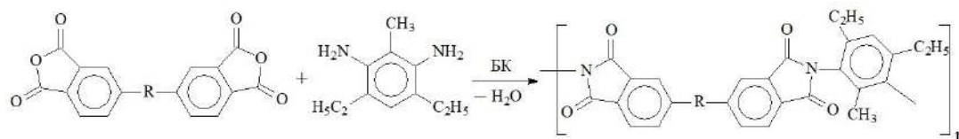
Рисунок 1. Схема синтеза ПИ на основе диамина ДЭТДА.
