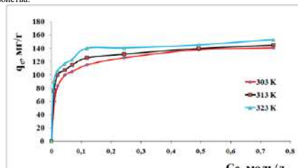
Рис 2. Изотерма сорбции ионов никеля (II) из искусственных растворов при различных температурах (время - 12 ч.)
