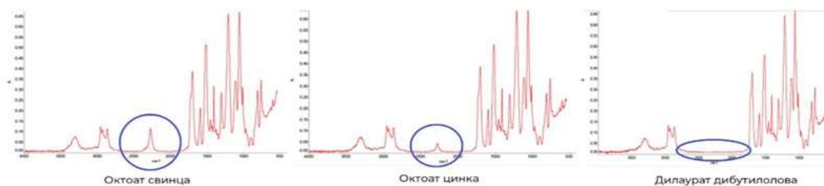
Рисунок 1. Сравнение пика изоцианатных групп при реакциях с различными катализаторами
