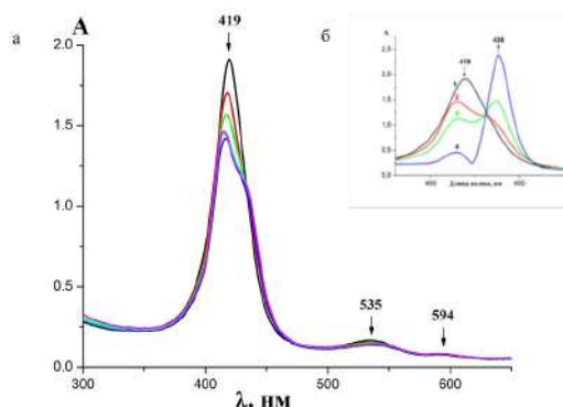
Рисунок 1. Изменение электронных спектров поглощения CoTnMPP при взаимодействии с P4VP, а) C(\text{CoTnMPP}) = 7,5 \cdot 10^{-6} моль/л; C(\text{P4VP}) = 4,5 \cdot 10^{-6} - 3,8 \cdot 10^{-5} моль/л; б) Соотношение CoTnMPP и P4VP 1:3 : 1-ЭСП CoTnMPP; 2- через 0 ч.; 3- через 2 ч.; 4- через 24 ч.
