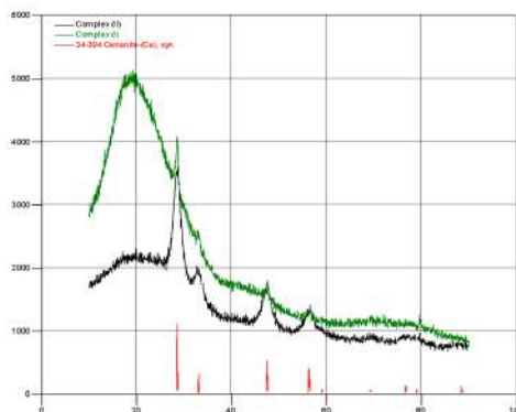
Рисунок 1. Рентгенограммы наноконкомпозитных полиимидных пленок с диоксидом церия.
