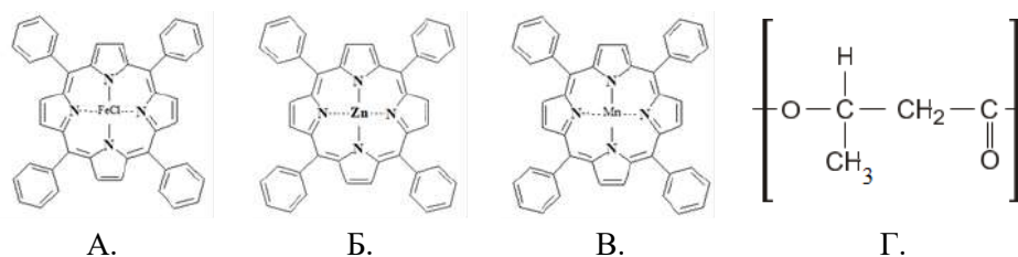
Рисунок 1. Металлопорфирины, использованные в работе: А – железо-порфирин (FeTPP); Б – цинк-порфирин (ZnTPP); В – марганец-порфирин (MnTPP); Г – мономерное звено биополимера поли-(3-гидроксипропирата) (ПГБ).
