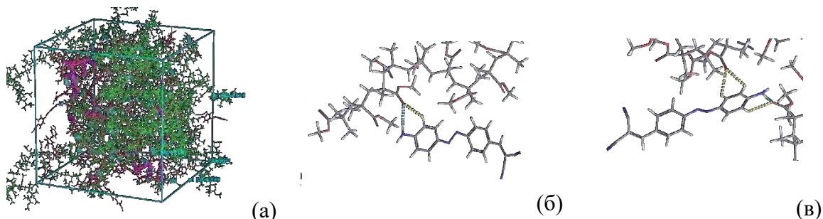
Рисунок. PMMA/AAB-DCV(30) в ячейке (а); водородные связи в материале (б, в).
