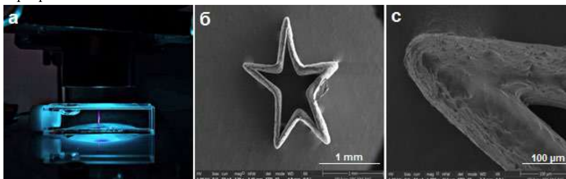
Рисунок 1. Фотоотверждение композиции из МГК, содержащей НАФ, в кювете: процесс фотоотверждения ИК-светом 975 нм (а), СЭМ фотография трехмерной микроструктуры в форме звезды длина 1 мм, высота 0,3 мм образующаяся в объеме жидкой фотоотверждаемой композиции (б, в).
