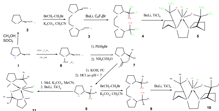
Схема. Синтез производных пропиона и титановых комплексов с их участием
