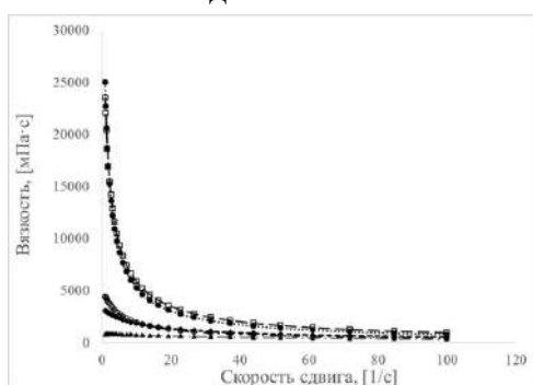
Рис.1 Зависимость вязкости 1% раствора гиалуроната натрия от состава растворителя: ●- H_2O ; □- NH_3 \cdot H_2O (33%)+НМП (2:1); ○- NH_3 \cdot H_2O (33%)+ ДМФА (2:1); ◆- NH_3 \cdot H_2O (10%)+НМП (2:1); ▲- NH_3 \cdot H_2O (10%)+ ДМФА (2:1)
