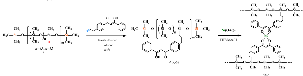
Рисунок 1. Общая схема получения координационно-сшитых полимеров
