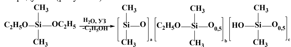
Рисунок 1. Схема ГПК диметилдиэтоксисилана под действием УЗИ.
