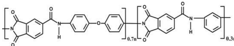
Рисунок 1. Структура полиамидоимида.
