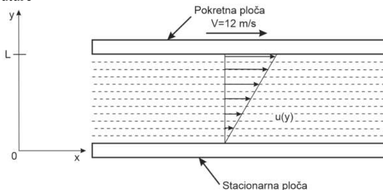
Slika 6. Šema za računski primjer 1 pravolinijskog kliznog ležišta
