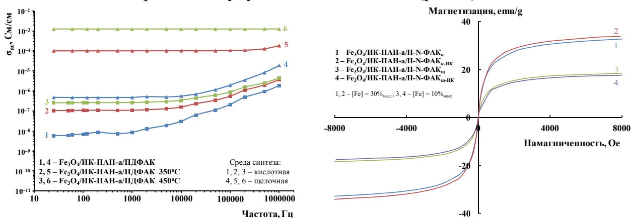
Рис. 1. Электропроводность и намагниченность насыщения нанокompозитов \text{Fe}_3\text{O}_4 /ИК-ПАН-а/ПДФАК.
