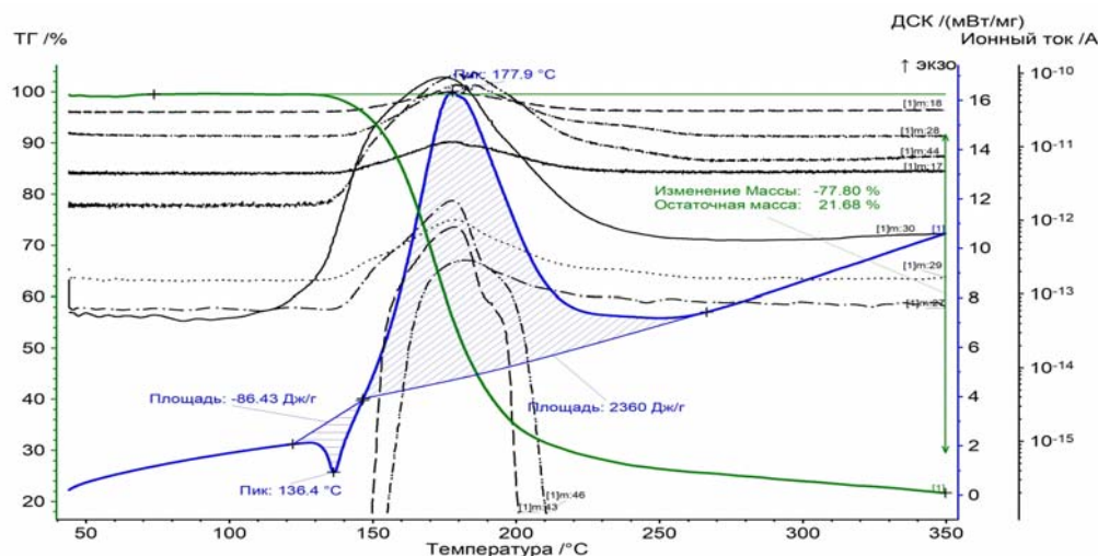
Рис. 2. Температурные зависимости ионных токов газообразных продуктов при скорости нагрева 10 °C/мин (величины m/e указаны над кривыми).
