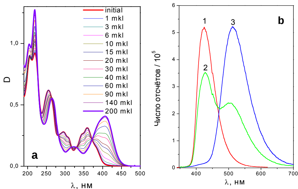
Рисунок 2. Поглощение (a) и люминесценция (b) типичного гелицена. (a) – изменение электронного спектра поглощения при последовательном добавлении \text{CF}_3\text{COOH} , (b) – спектры люминесценции при разных концентрациях кислоты.
