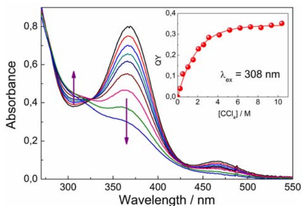
Стационарный фотолиз раствора комплекса \text{Ni}(\text{dsepi})_2 в \text{CCl}_4 светом \text{XeCl} эксилампы (308 нм). Во вставке – зависимость квантового выхода фотолиза комплекса от концентрации \text{CCl}_4 в ацетонитриле.
