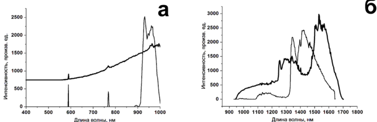
Рис. Спектры излучения пламени H 2 /D 2 + воздух тонкая линия 40% H 2 + воздух, толстая линия - 17% D 2 + воздух: (а) – 400 -900 нм; (б) 900-1650 нм.
