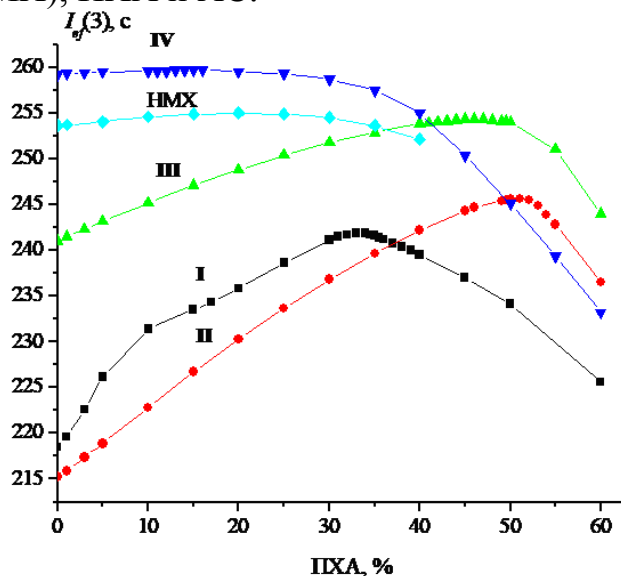
Рис. 1. Зависимость I_{\text{ef}}(3) состава « I–IV или HMX + АС + ПХА» от доли ПХА в смешанном наполнителе при объемном содержании АС 18%.
