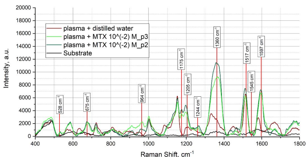
Рисунок 1. Спектры КРС от плазмы, разведенной дист. водой и плазмы, разведенной MTX концентрацией 10^{-2} М.
