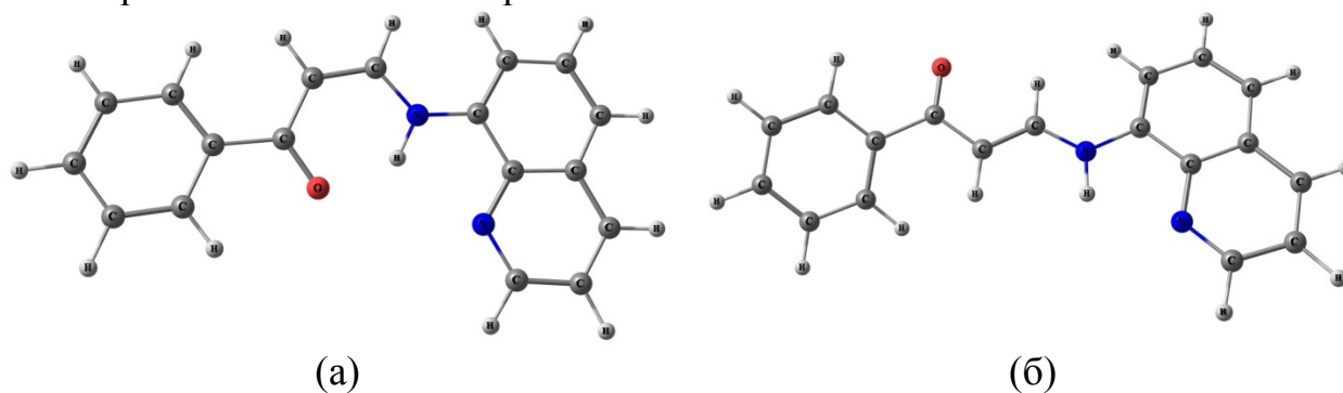
Рис. 1 Оптимизированная геометрия cis - (а) и trans - (б) изомеров, рассчитанные методом DFT (CAM-B3LYP/ def2-TZVP) без учета растворителя
