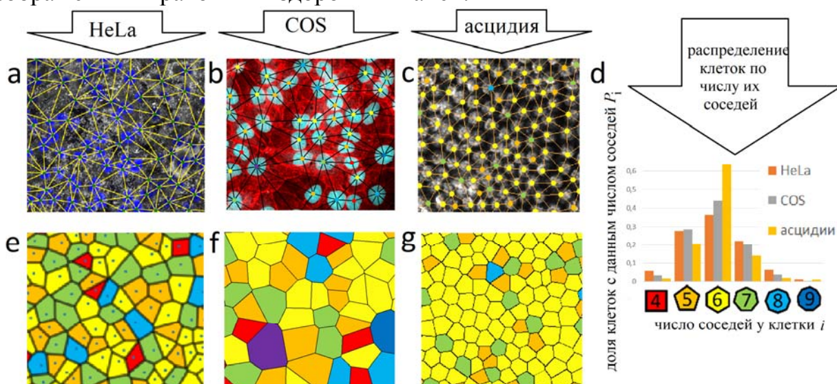
Рис. 1. Микрофотографии монослоев эпителия HeLa (a,e), COS (b,f), асцидий (c,g) с наложенными триангуляцией Делоне (верхняя строчка) и разбиением Вороного (нижняя строчка панелей).
