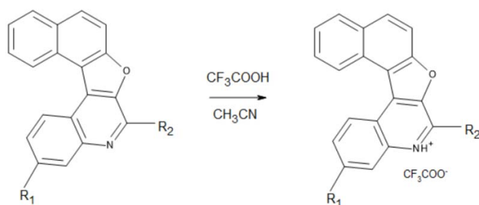
Рисунок 1. Люминесцентные гелицены. R_1 = \text{Br}, \text{OMe} . R_2 = \text{MeOPh}, \text{Me}, \text{Ph}, \text{CF}_3\text{Ph} .
