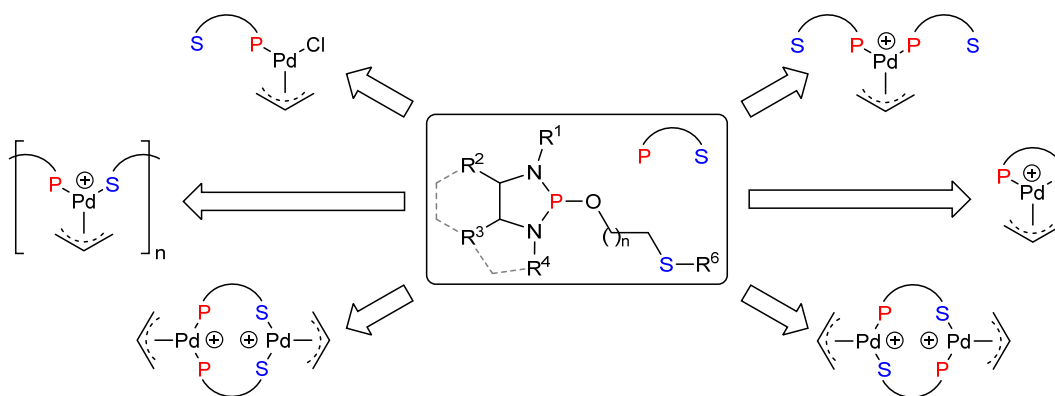
Рисунок 1. Координационное поведение диамидофосфитных лигандов с тиоэфирными фрагментами.
