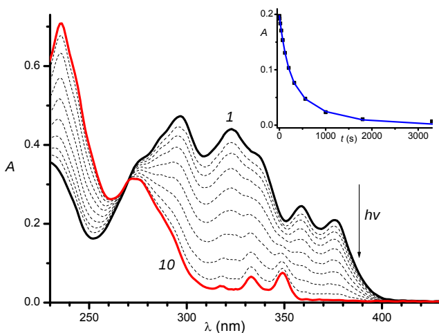
Рис. 1. Спектральные изменения при облучении воздушно-насыщенного раствора диады D11B ( 6.8 \times 10^{-6} M) светом с длиной волны 372 нм, интенсивность 1.8 \times 10^{-10} эйнштейн \text{см}^{-2} \text{с}^{-1} , время фотолиза (1) – (10) 0 – 3300 с. Вставка: кинетика изменения оптической плотности на длине волны 372 нм, экспериментальные точки и аппроксимирующая кривая.
