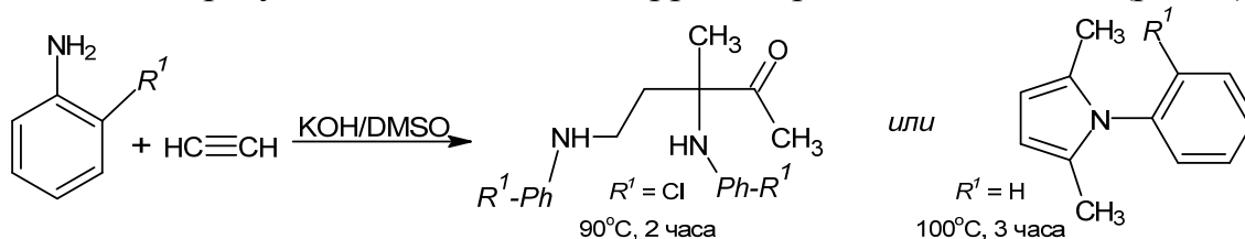
Рисунок 1. Образование 3,5-бис(галоанилин)-3-метилпентан-2-она
