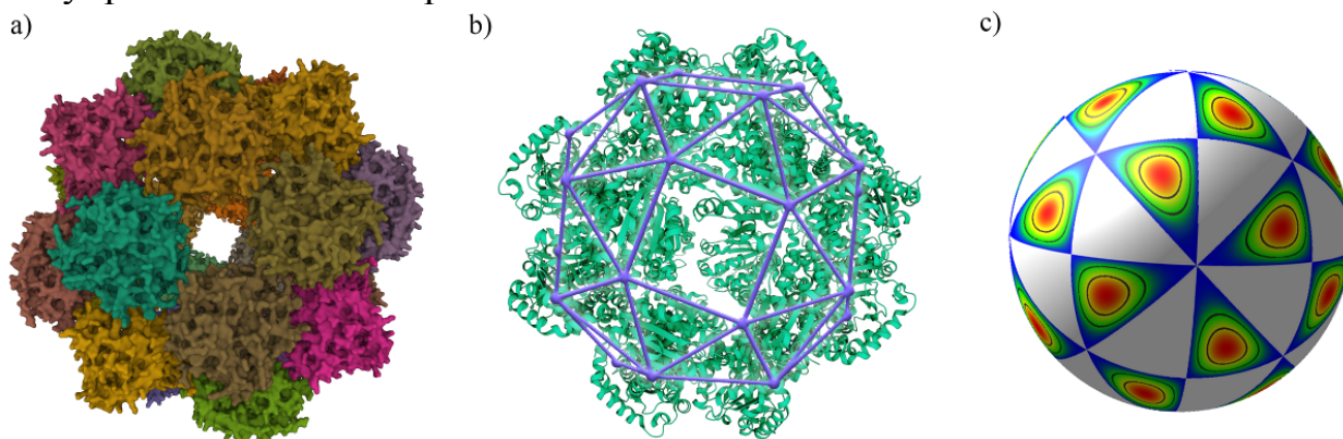
Рис. 1 (a-b) Модель нанокластера, состоящего из 24х белков \alpha -ТТР, с наложенным курносым кубом (с) Волна плотности, соответствующая данной упаковке.
